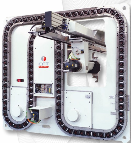
CTA 40 HS 120 utensili/tools
