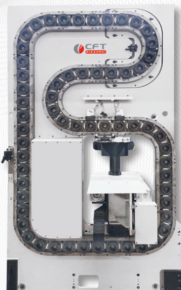
CTA 50 HS 46 utensili/tools
