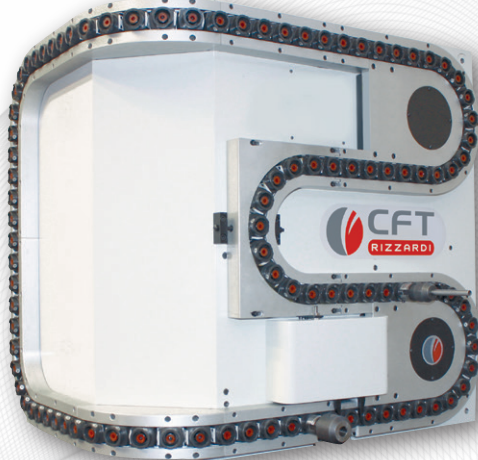
CTA 40 HSL 65 utensili/tools
